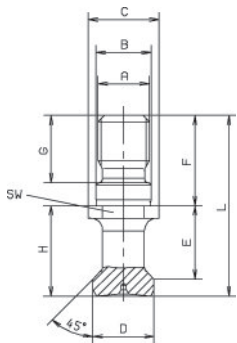
A 34 Anzugsbolzen für Spannköpfe
